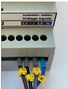
Bild 7 - Position des Steckers für die Drähte L1, L2, L3, N.
