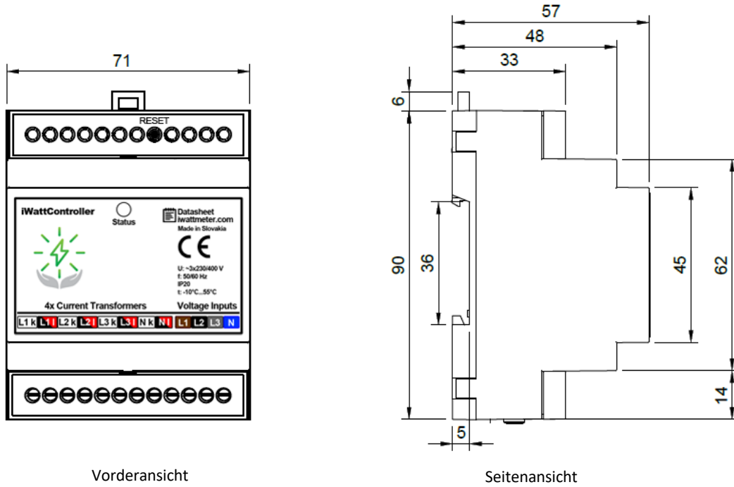
Bild 1 – Gehäuseabmessungen des iWattController.
