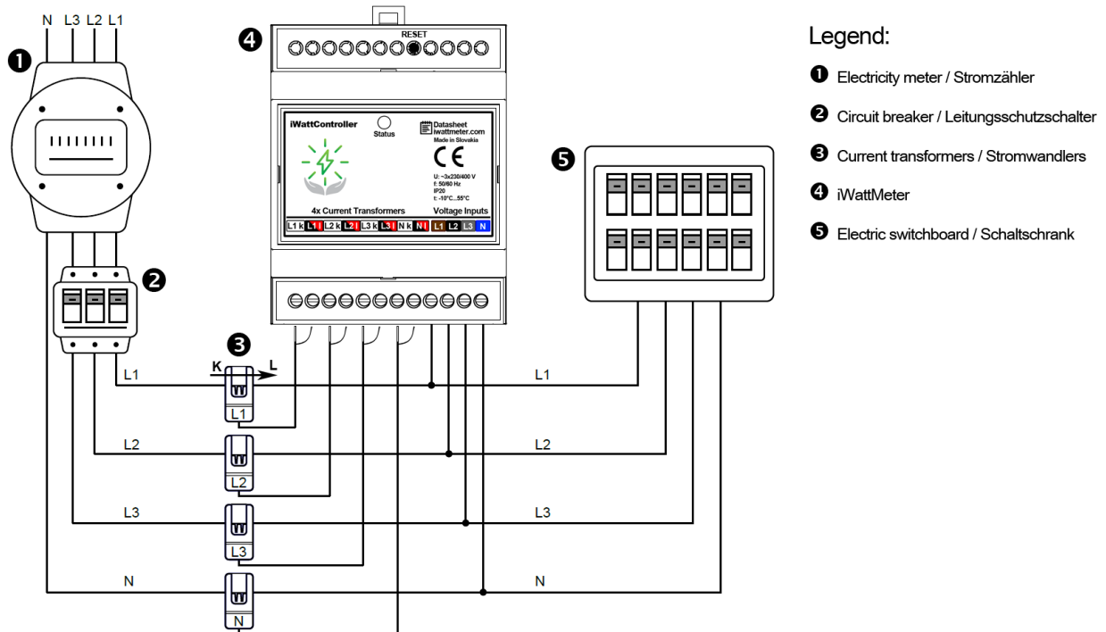
Bild 2 - Schaltplan des iWattController
