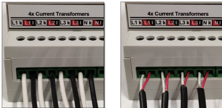
Bild 9 - Die Farben der Kabel müssen mit den Farben auf der Verpackung übereinstimmen.
