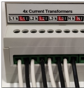
Bild 8 - Eingelegte Drähte der Stromwandler.
